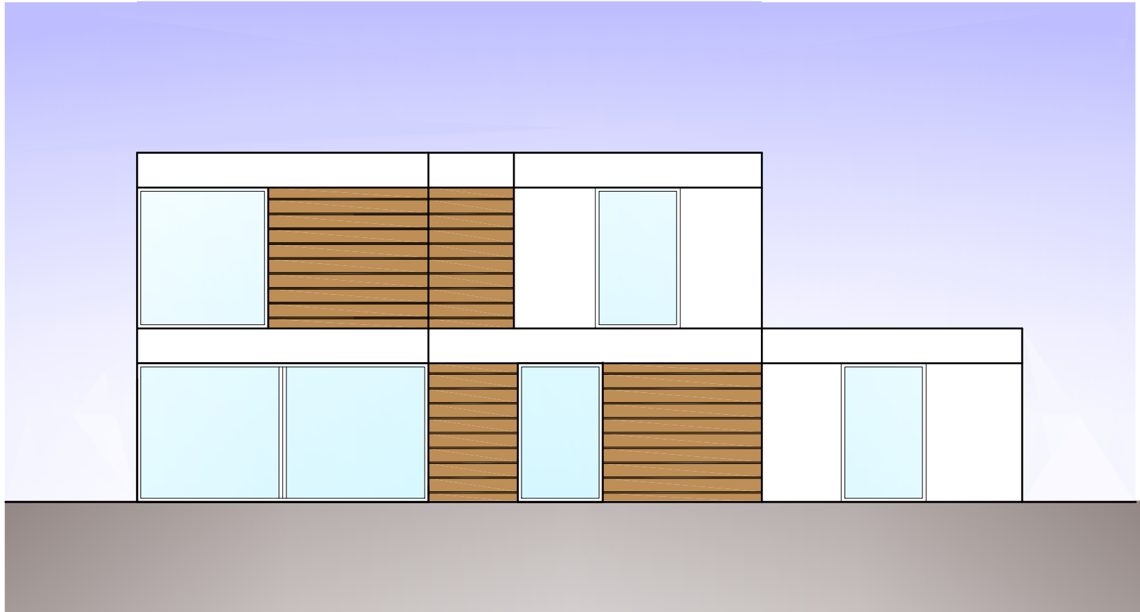
ALZADO SUR ESCALA 1.100
