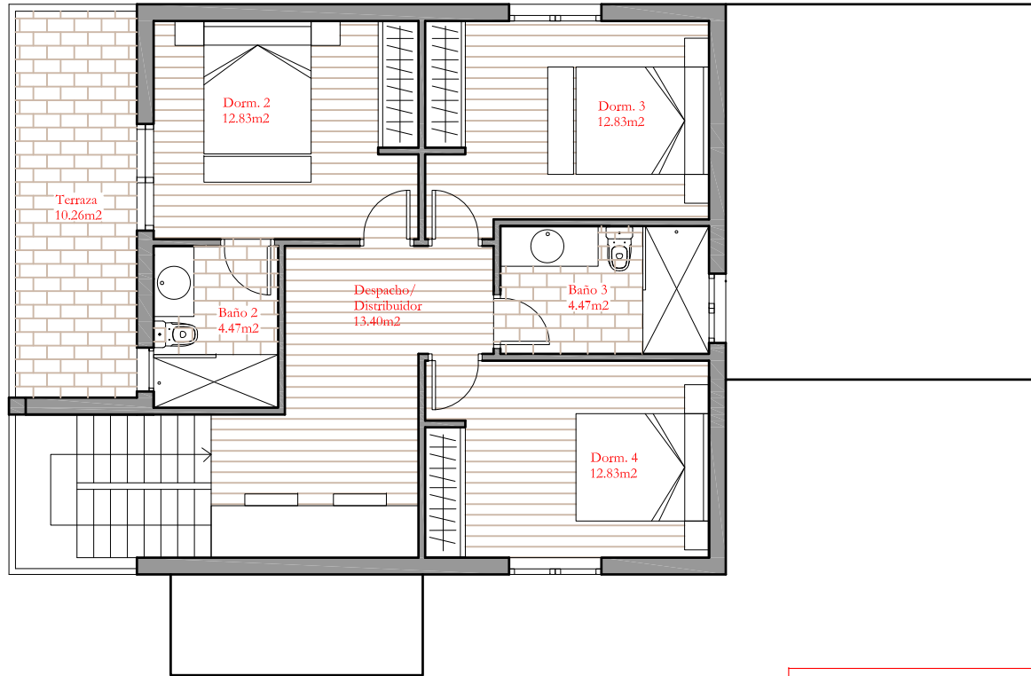
PLANTA PRIMERA ESCALA 1.100
