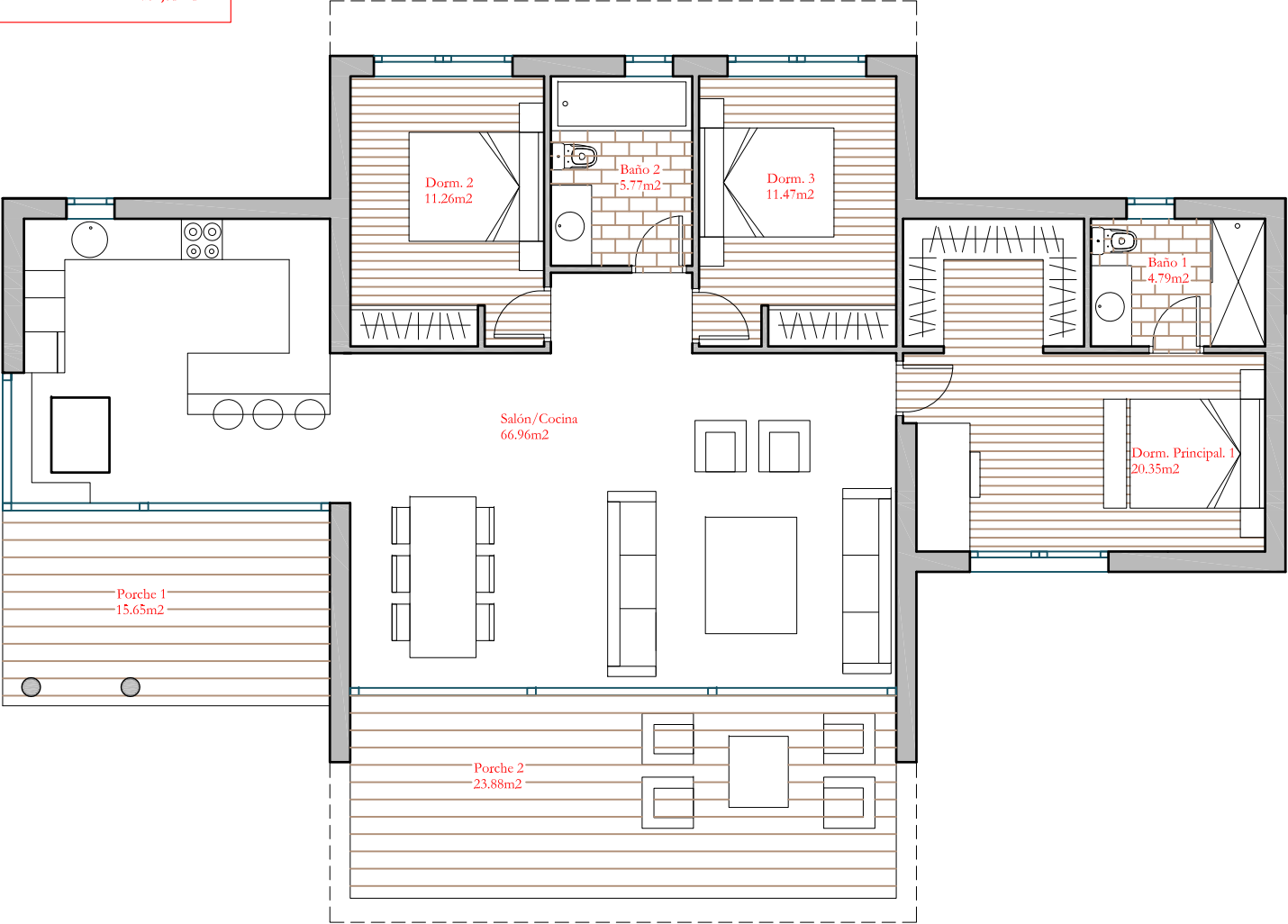
PLANTA BAJA ESCALA 1.100
